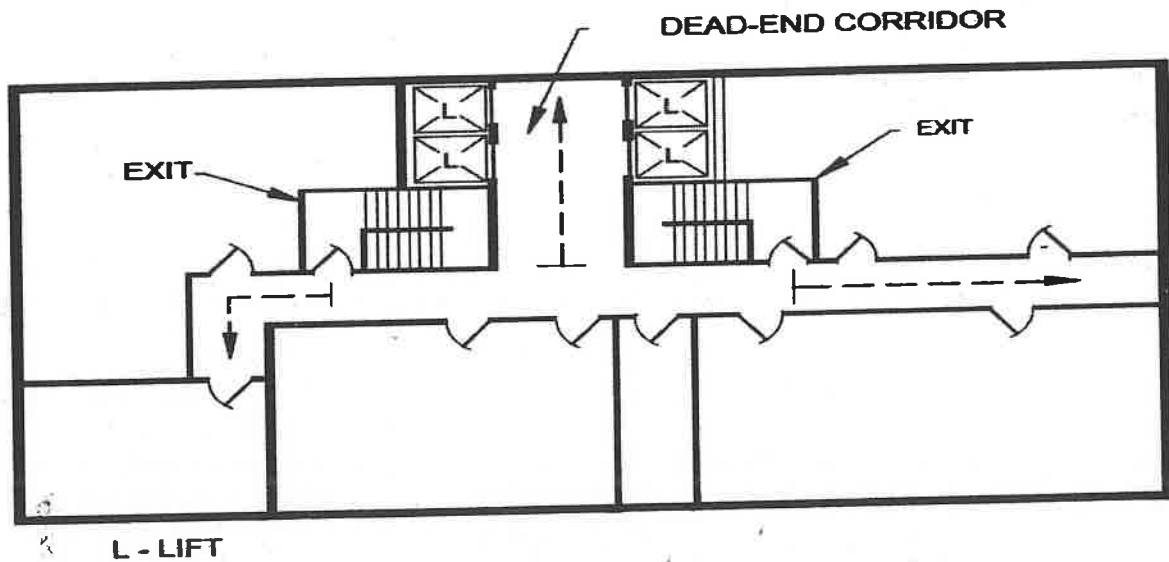
FIG. 9 DEAD END CORRIDOR
